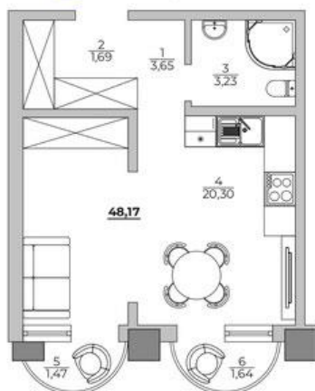
План на апартаментите
