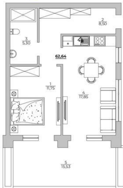
План на апартаментите
